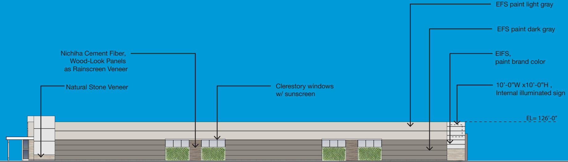
RIGHT ELEVATION
