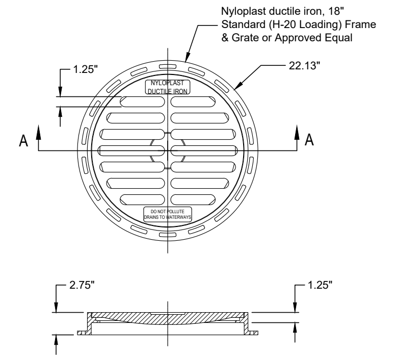
18" Frame & Grate Details Scale: None
